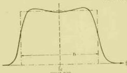
ציר 2. עקום הסלקטיביות של חקלט טיפוסי
